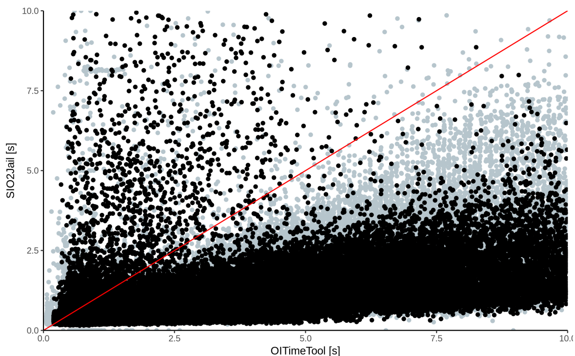
Rysunek 4.5: Rzeczywisty czas sprawdzania za pomocą SIO2Jail w zależności od czasu sprawdzania za pomocą OITimeTool. Każdy punkt odpowiada jednemu uruchomieniu pewnego zgłoszenia na pewnym teście. Wyszarzone punkty ( err ) odpowiadają niepoprawnym zgłoszeniom.
