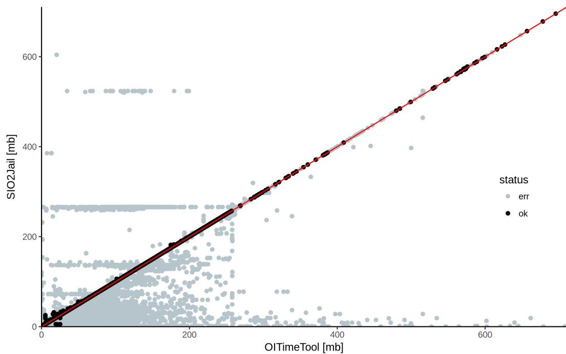
Rysunek 4.3: Zużycie pamięci zmierzone za pomocą SIO2Jail w zależności od zużycia zmierzonego za pomocą OITimeTool. Każdy punkt odpowiada jednemu uruchomieniu pewnego zgłoszenia na pewnym teście. Wyszarzone punkty ( err ) odpowiadają niepoprawnym zgłoszeniom.
